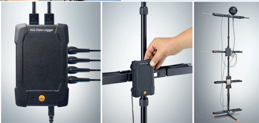
Per una misura affidabile, fissare semplicemente tutte le sonde necessarie al cavalletto.
