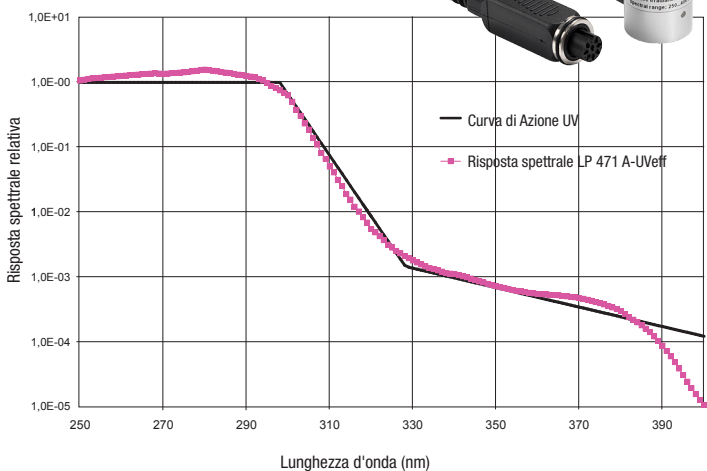
Curva di risposta tipica della sonda LP471A-Uveff:
